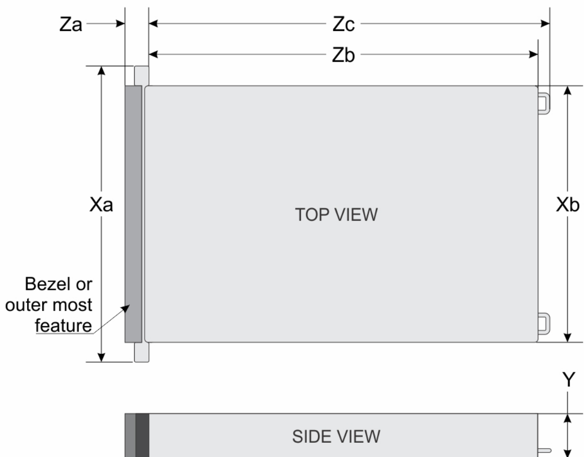
그림 48 . 새시 크기
