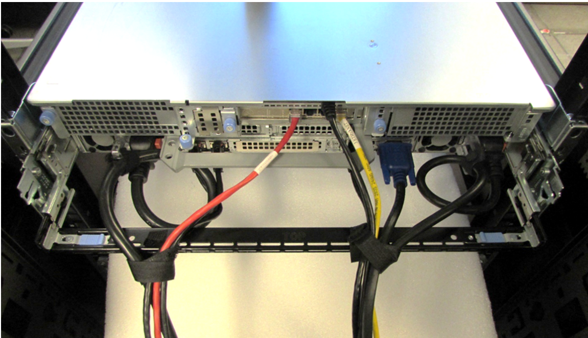
그림 39 . 케이블 연결된 SRB(Strain Relief Bar)
