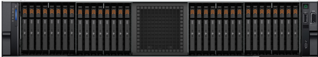
그림 6 . 32개의 EDSFF E3.S 전면
