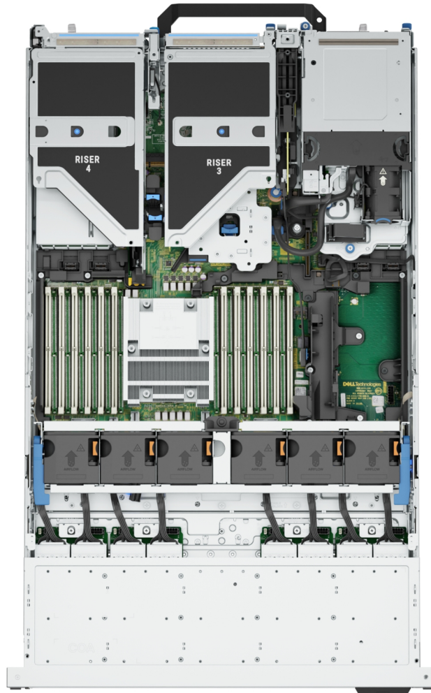
그림 17 . 라이저 + 4개의 후면 EDSFF E3.S가 있는 시스템의 내부
