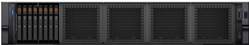
그림 8 . 8 x EDSFF E3.S의 전면
