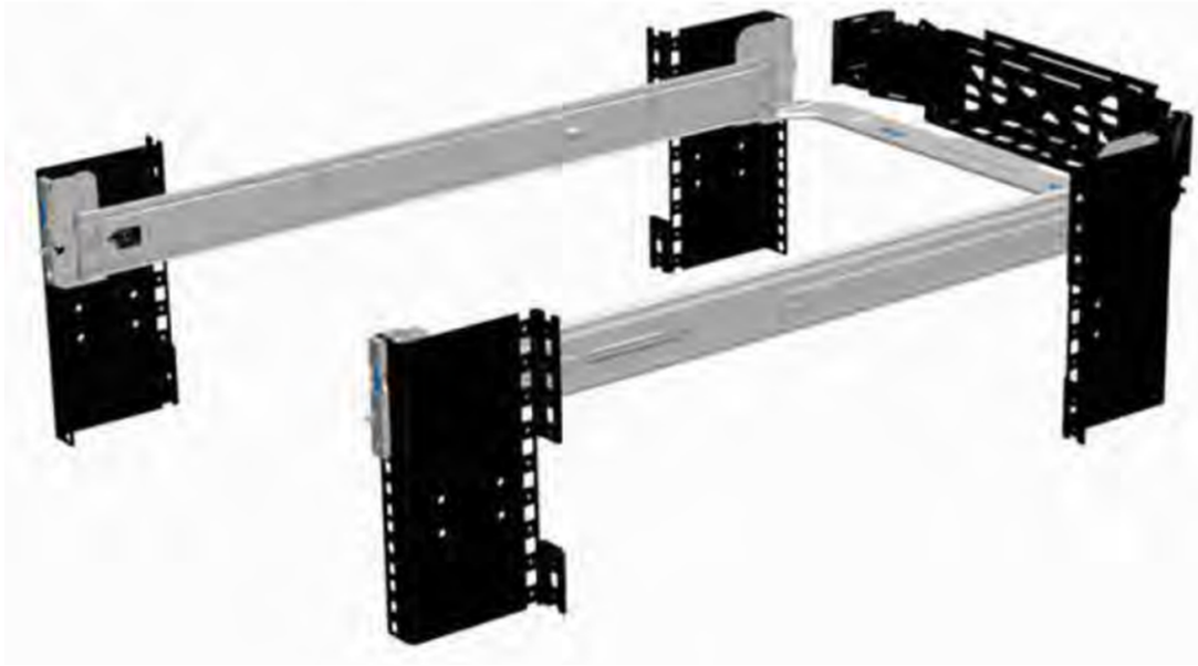
그림 34 . 슬라이딩 레일과 CMA 옵션
