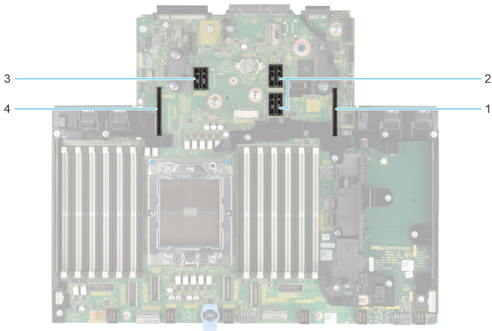
그림 18. 확장 카드 라이저 슬롯 커넥터
