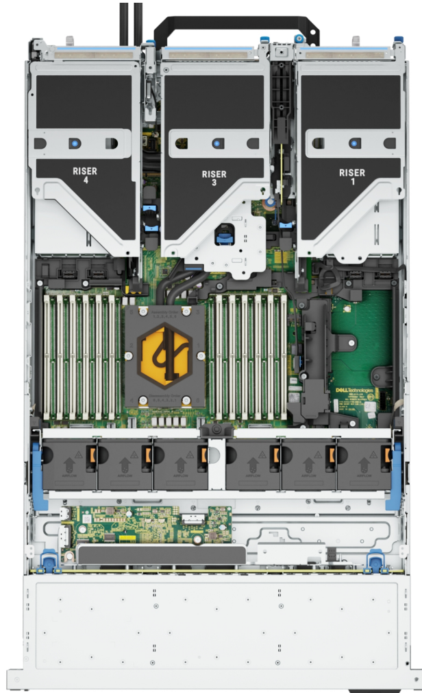
그림 16 . 프로세서 액체. 냉각 모듈이 있는 시스템 내부
