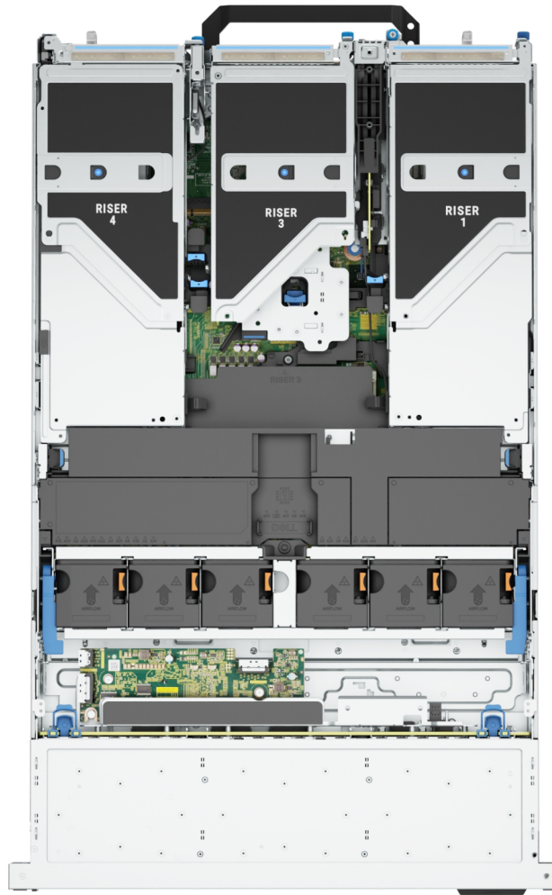
그림 15 . FL(Full Length) 라이저 및 GPU 덮개가 있는 시스템 내부
