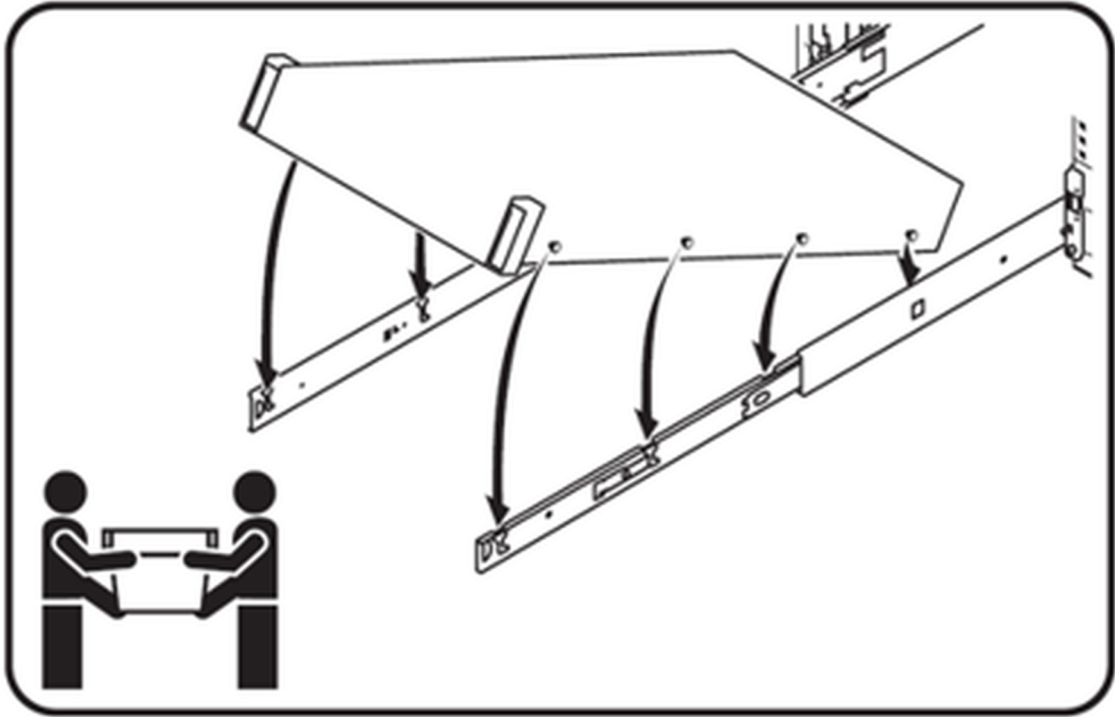
그림 40 . 드롭인 슬라이딩 레일에 시스템 설치
