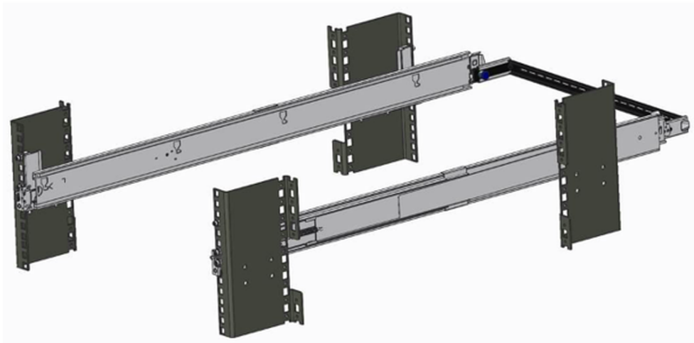
그림 35 . 슬라이딩 레일과 SRB 옵션
