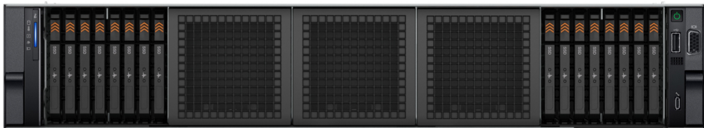
그림 7 . 16 x EDSFF E3.S의 전면
