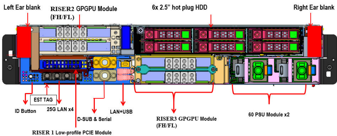
図 11. XR12 背面アクセス シャーシの背面図
