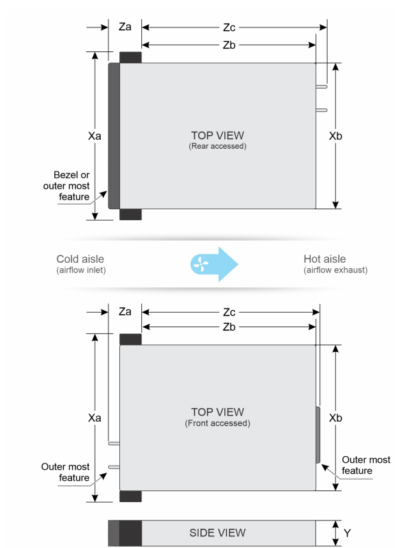
図 50. 背面アクセス（上）と前面アクセス（下）の XR11 シャーシ寸法
