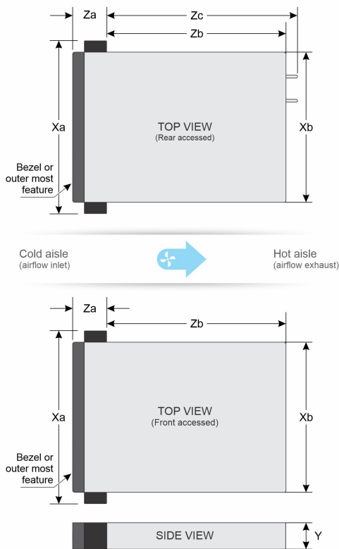
図 51. 背面アクセス（上）と前面アクセス（下）の XR12 シャーシ寸法
