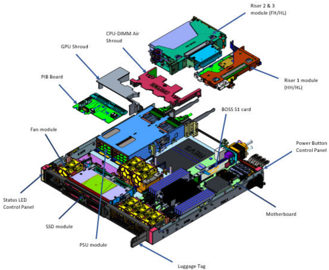
図 13. XR11 前面アクセス シャーシ内部の分解図 (背面から前面)
