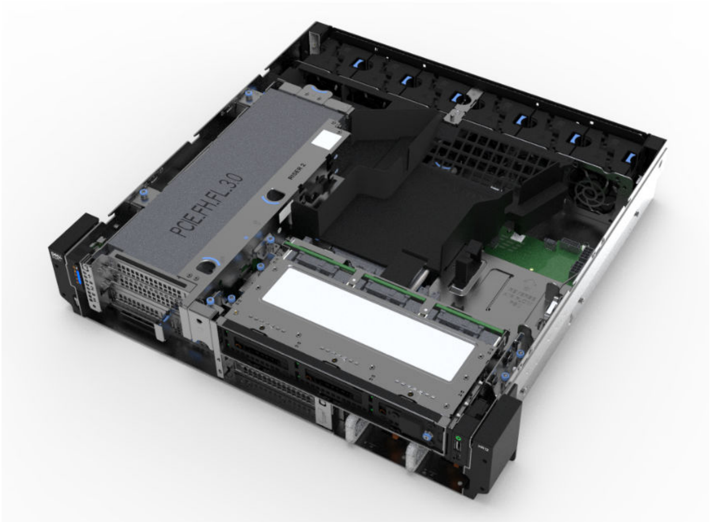
図 16. XR12 前面アクセス シャーシ内部の前面図 (ベゼルなし)
