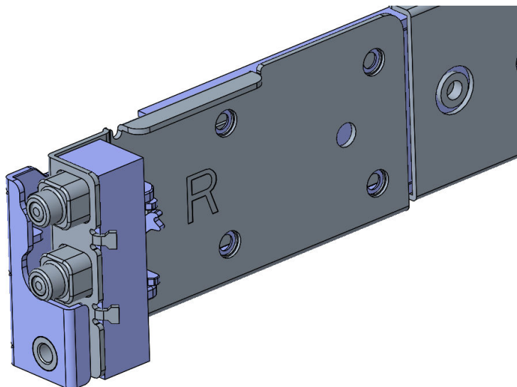
図 38.4 ポスト丸穴または角穴ラック用の XR11 と XR12 スタブインスライド レール取り付けインターフェイス
