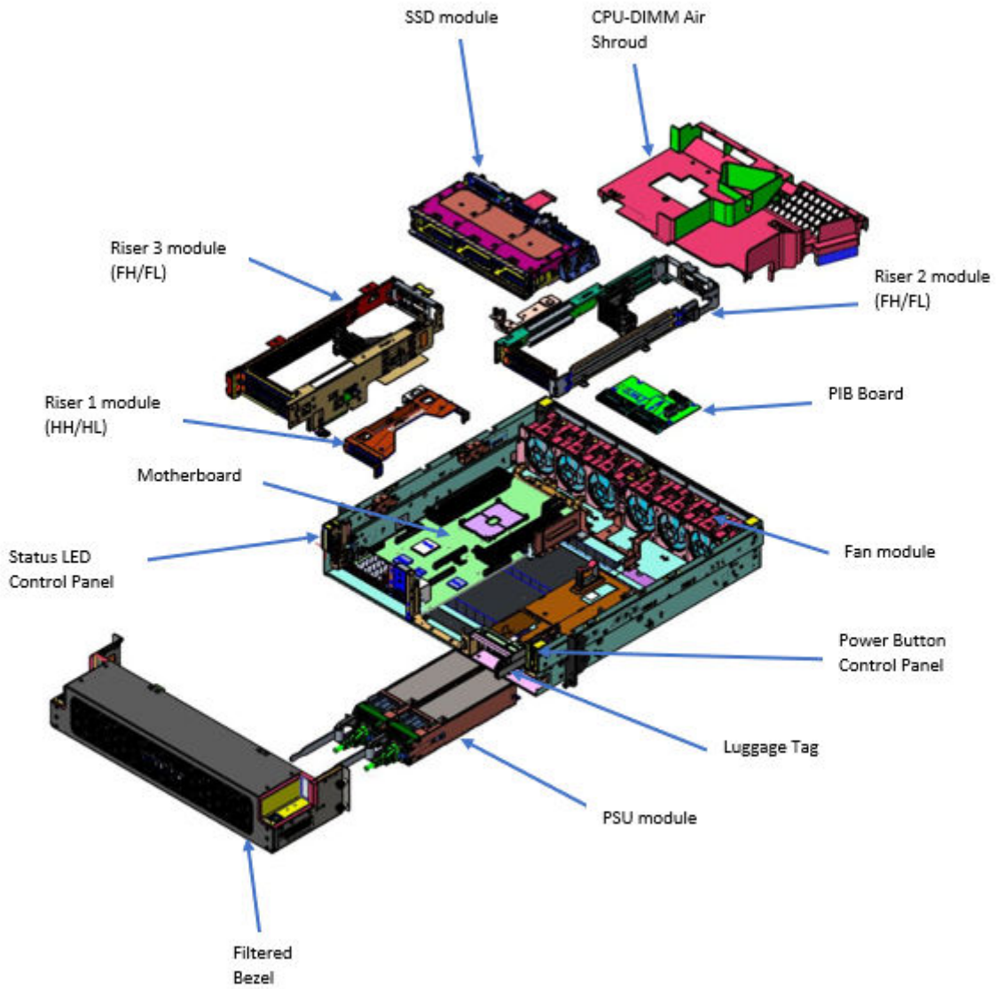
図 17. XR12 前面アクセス シャーシ内部の分解図
