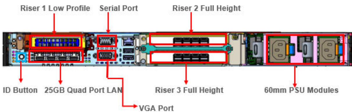
図 9. XR11 背面アクセス シャーシの背面図
