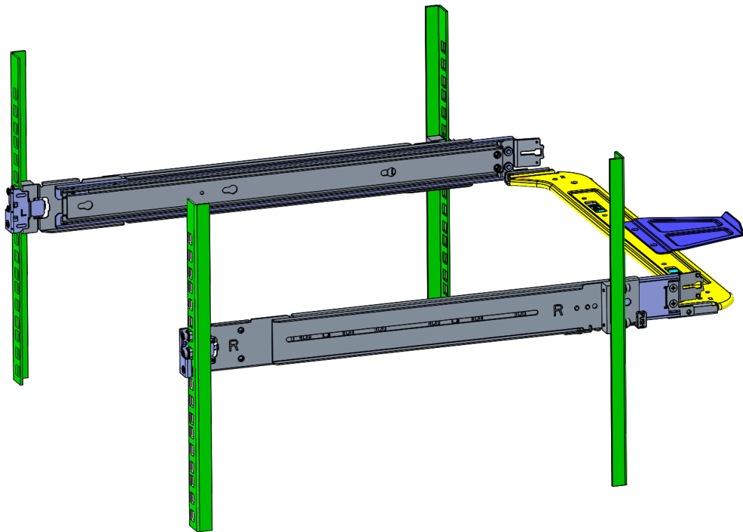
図 43. オプションの SRB 付きのスライドレール
