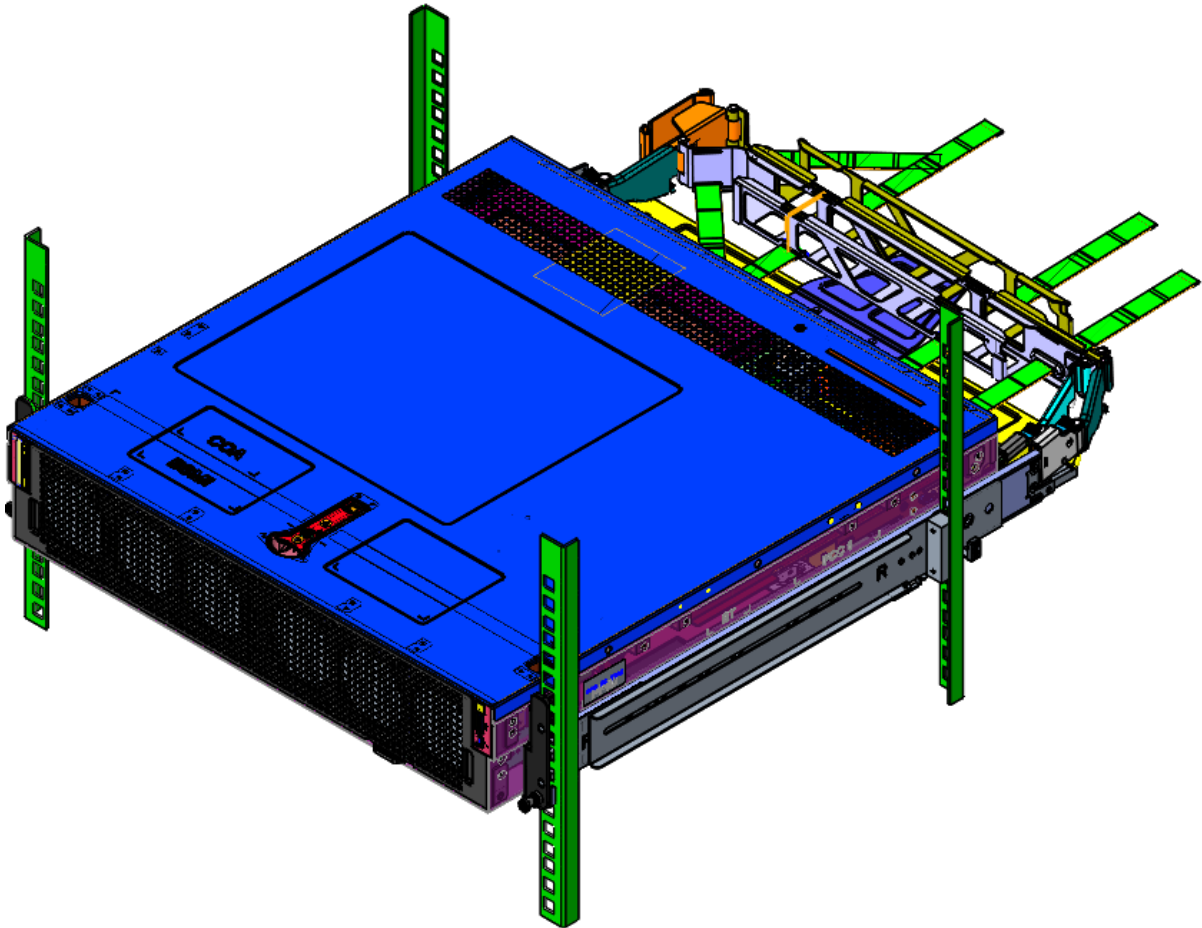
図 40. 4 ポスト ラックの CMA を使用したスライド レールに取り付けた XR12
