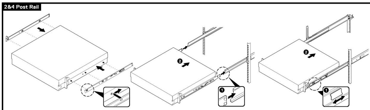
図 35. システムをスタブイン スライド レールに取り付ける
