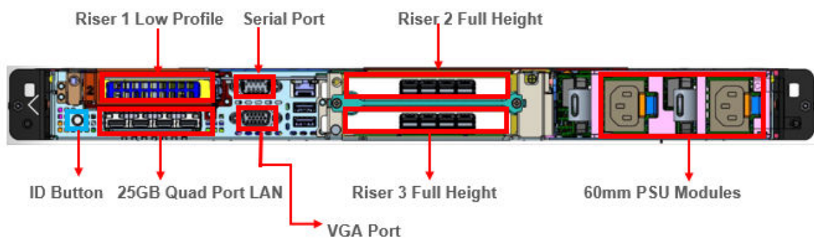
図 1. XR11 前面アクセス シャーシの前面図
