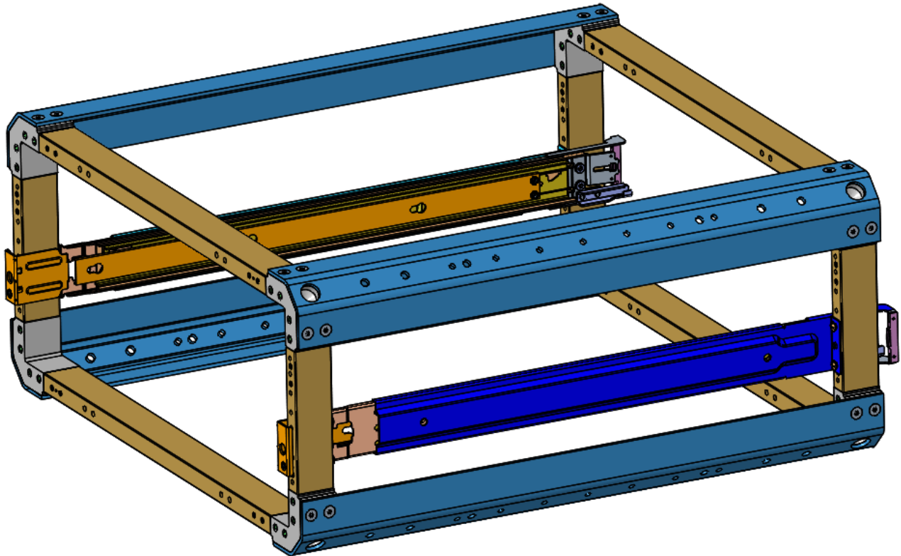
図 41. Pelican ケース フレーム内の XR11 と XR12 の輸送ケース レール
