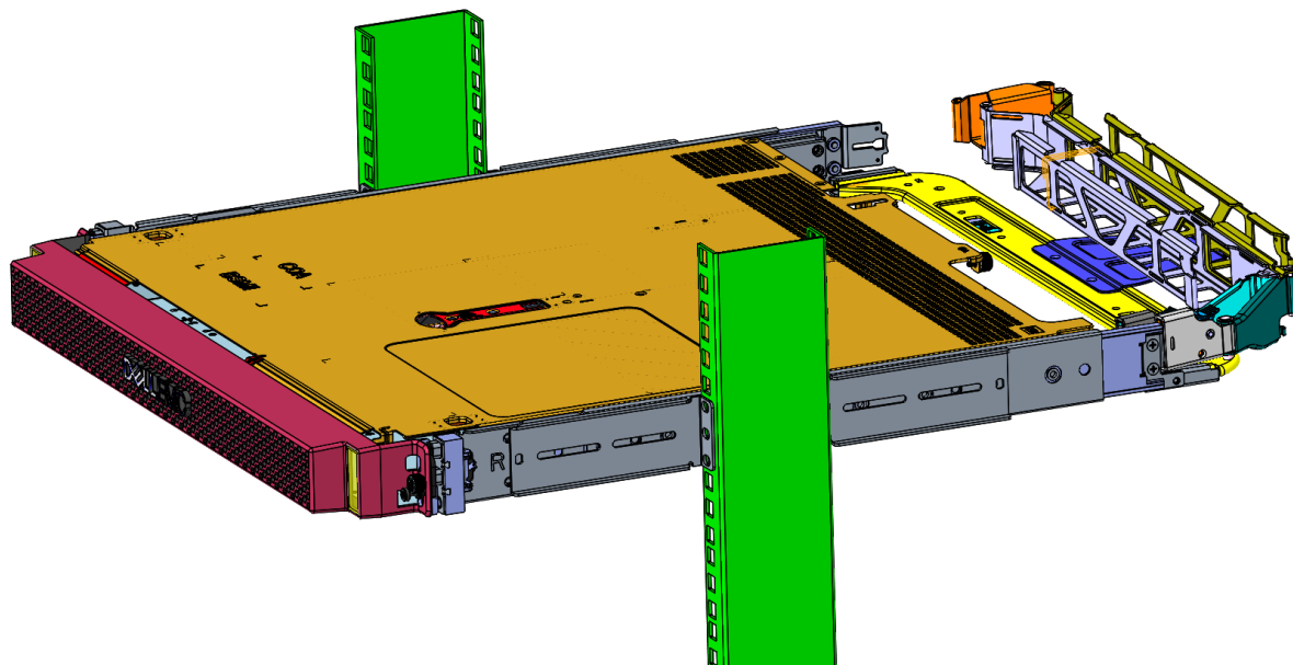
図 36. 2 ポスト センターマウント構成でスライド レールに取り付けられた XR11
