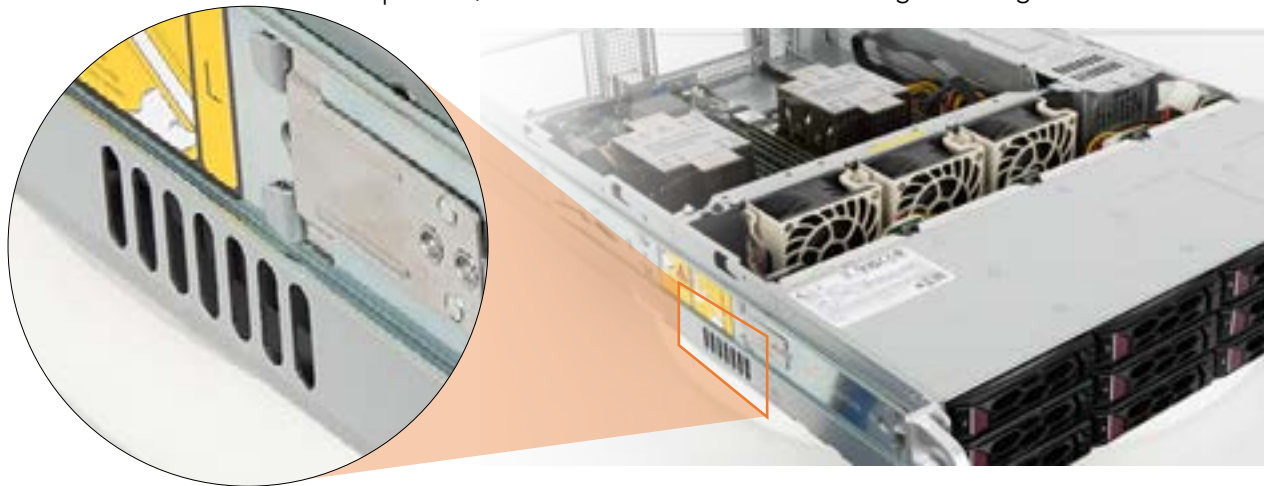
Figure 3 : Entrées d'air du châssis du Supermicro SYS-621C-TN12 que nous avons testé, qui peuvent permettre à l'air préchauffé de l'allée chaude de circuler à travers les composants du serveur. Source : Principled Technologies.
