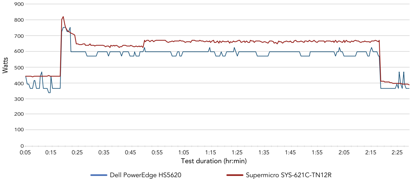
Figure 9 : Consommation électrique, en watts, du Dell PowerEdge HS5620 et du Supermicro SYS-621C-TN12 au cours du deuxième scénario, où les serveurs ont exécuté une charge applicative à virgule flottante avec un ventilateur désactivé sur chaque serveur. La charge applicative a commencé à 0:15 et s’est terminée à 2:15. Source : Principled Technologies.
