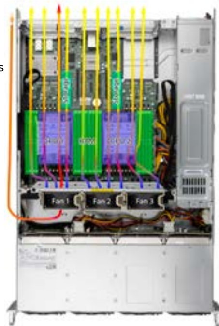
Figure 1 : Disposition de la carte mère du Supermicro SYS-621C-TN12 que nous avons testé. Nous avons ajouté des étiquettes de composants et des flèches indiquant la direction du flux d'air en provenance des ventilateurs. L'air plus froid est indiqué par des flèches bleues et violettes, et l'air plus chaud est indiqué par des flèches rouges, orange et jaunes. Source : Principled Technologies.
