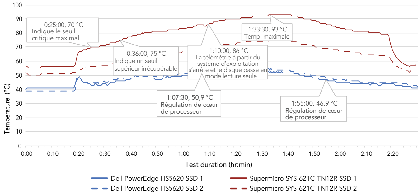
Scénario 3 : Températures des disques SSD
